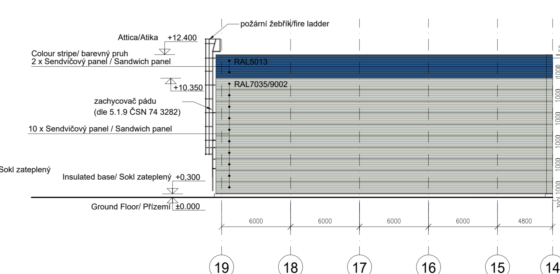
POHLED ZÁPADNÍ / WEST ELEVATION
