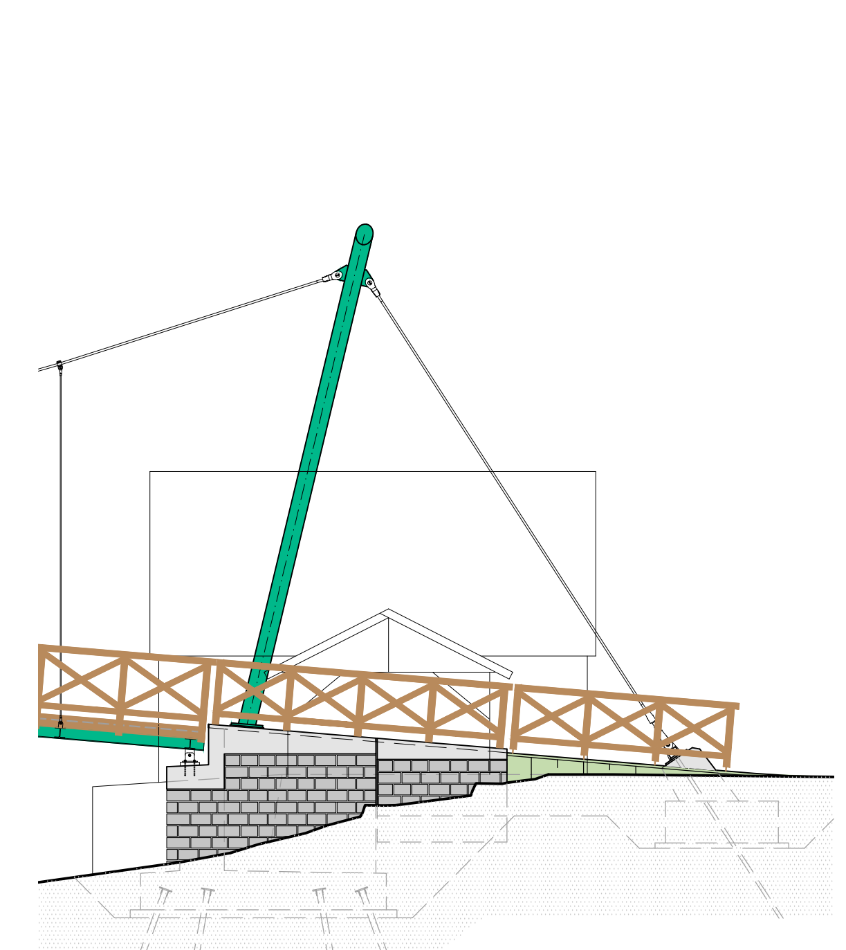
BOČNÍ POHLED NA OPĚRU 20 1:100
